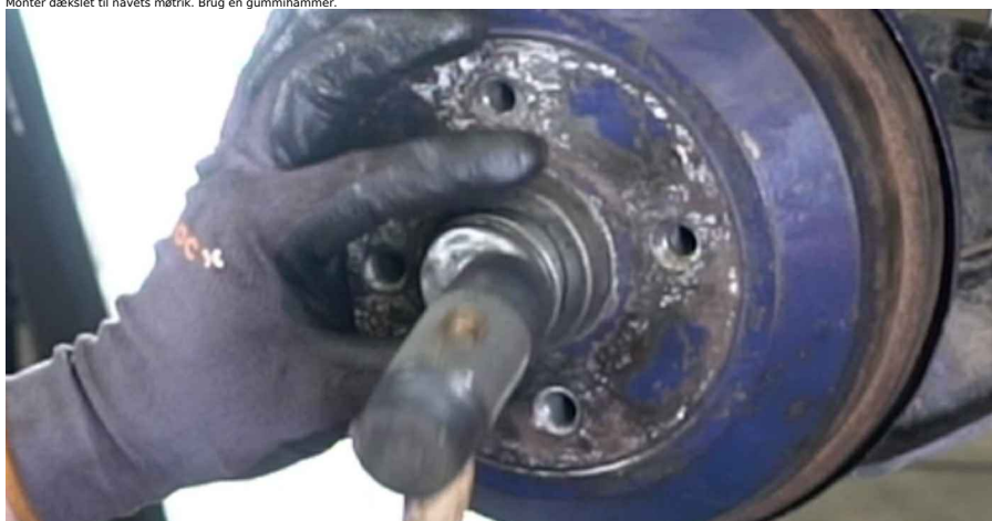
35 Behandel overfladen hvor hjulremmen berører bremsetromlen. Brug keramisk fedt.
