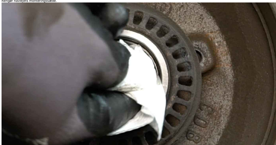
15 Fjern den indre skal af hjullejet fra bremsetromlen. Brug en universal aftrækker.
