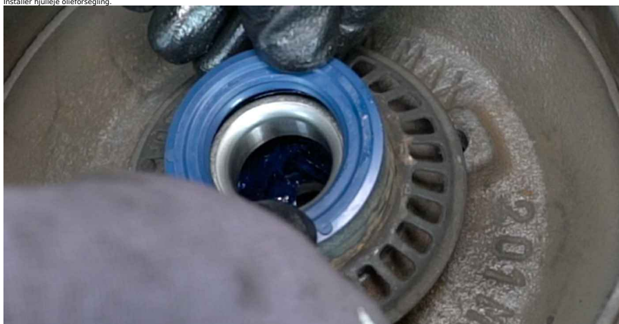
23 Behandl akseltappen. Brug universal rengøringsmiddel. Brug lelefedt.
