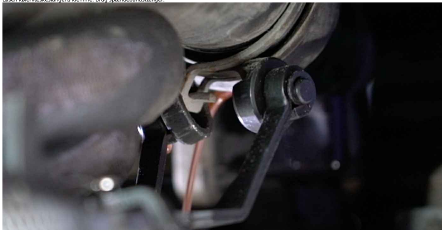
8 Frigør kølervæskeslangen.
